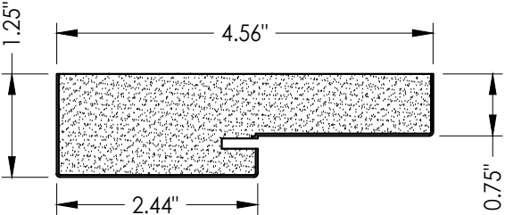
1 COMPOSITE JAMB
